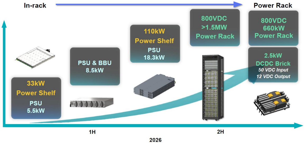
圖 10：光寶科隨 GPU 伺服器電源架構演進，持續提供解決方案
